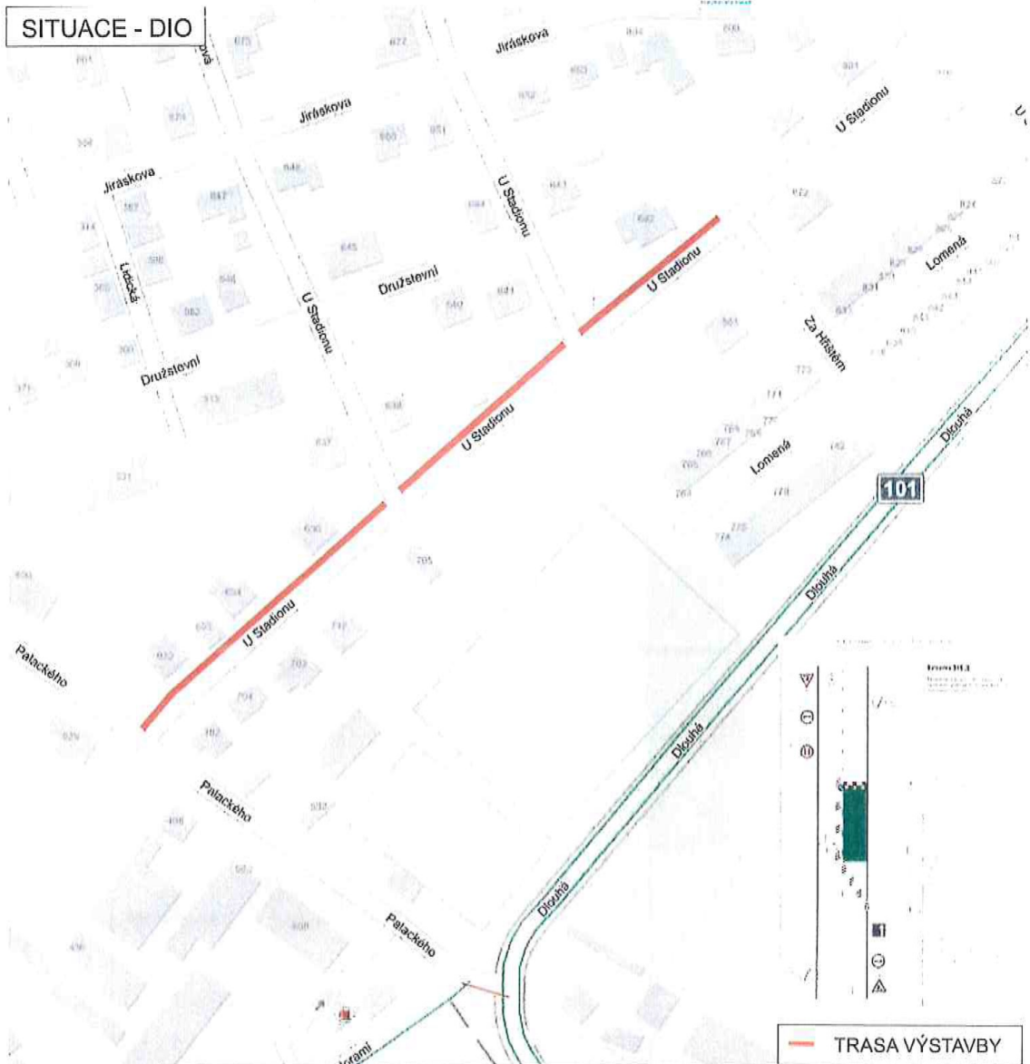
DOPRAVNÍ OPATŘENÍ - POSUVNÉ PRACOVNÍ MÍSTO - DLE TP66 - DLE SCHÉMATU B/5.2
