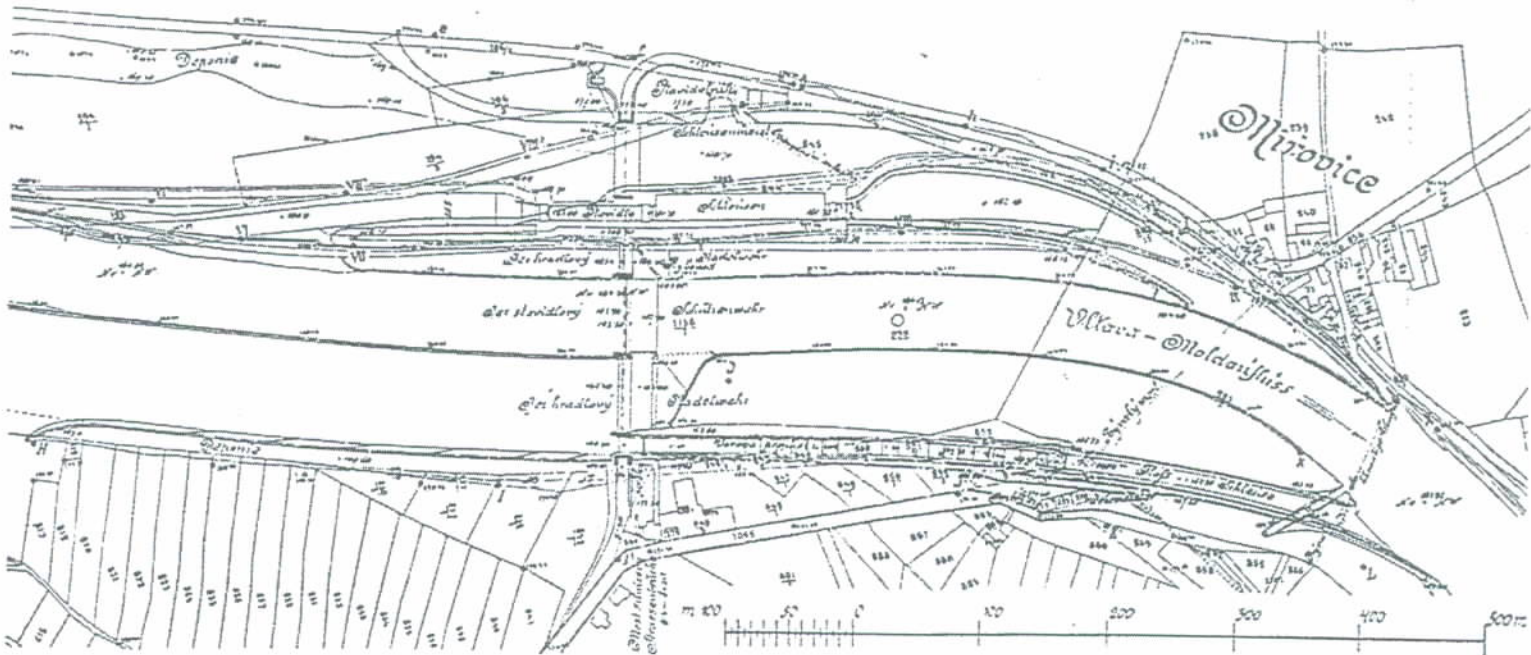
Obr. 1. Polohopis mostu a zdymadla u Mifovic a Veltrus.
